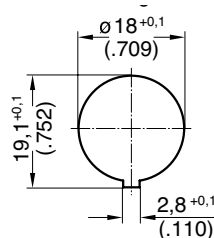
Montage- ausschnitt
