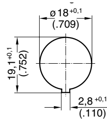
Montage- ausschnitt
