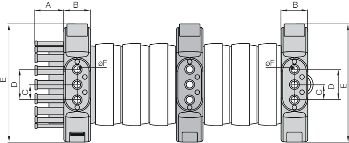
Anschlusselement mit Zugentlastung TR.XX.01
