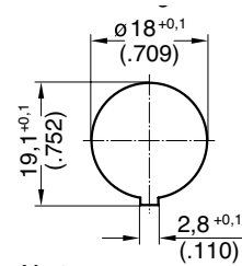
Montage- ausschnitt
