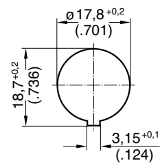
Montage- ausschnitt
