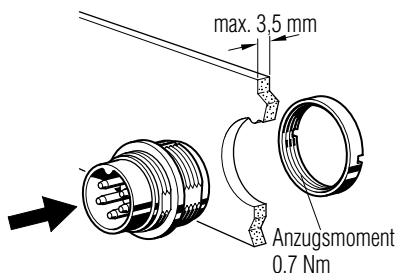
Montageausschnitt
