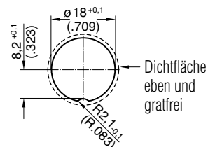
Montageausschnitt
