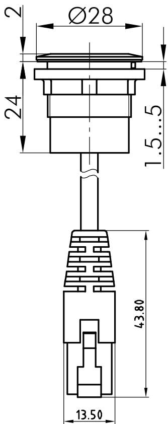
RRJ_RJ45
