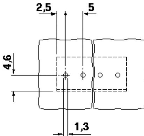
Bohrplan
