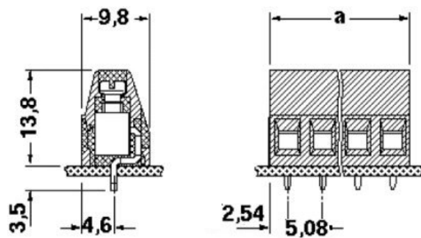
Maßzeichnung
