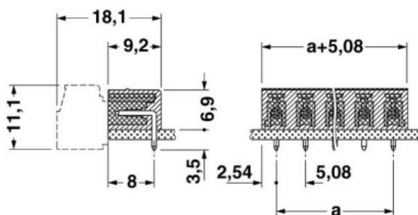
Maßzeichnung
