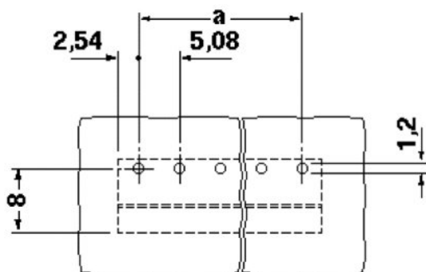
Bohrplan
