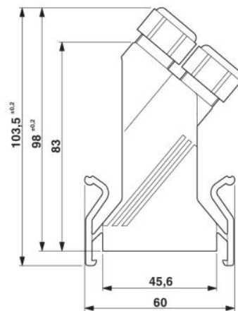
D-SUB Tüllengehäuse
