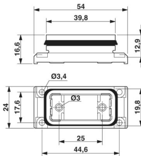
D-SUB Anbaurahmen
