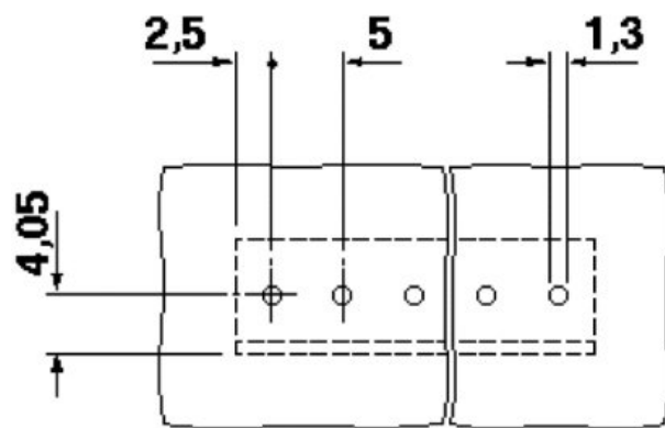
Bohrplan
