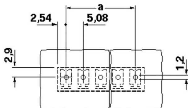
Bohrplan
