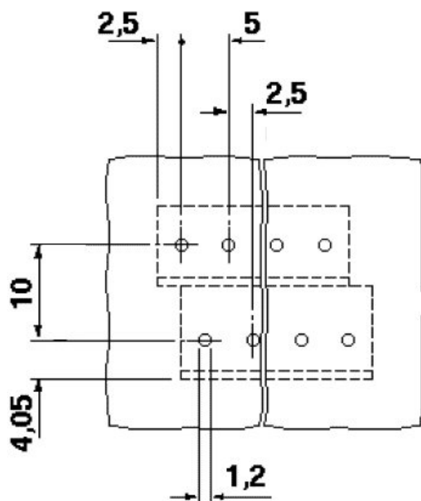
Bohrplan
