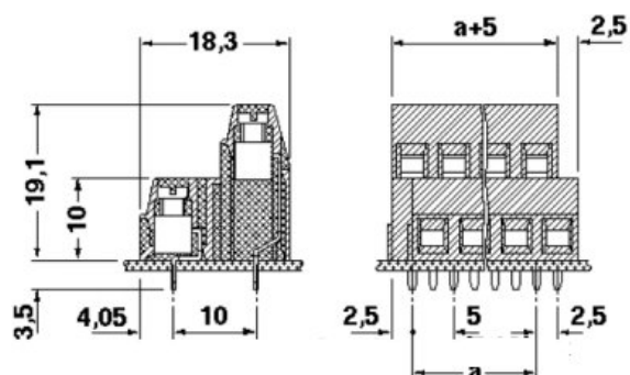
Maßzeichnung
