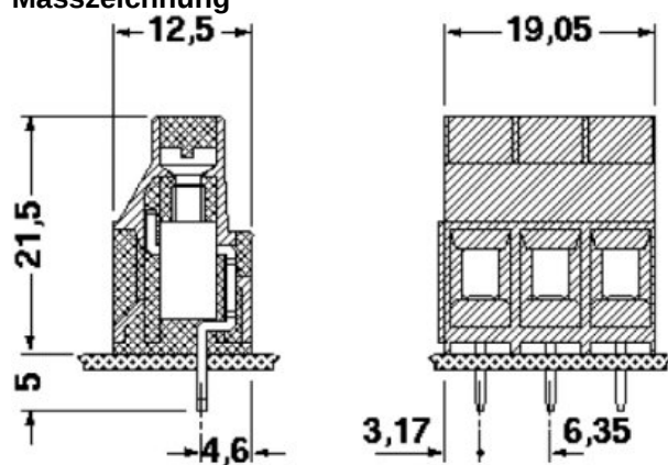
Masszeichnung
