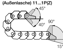
11...2P(Z) Festpunkt mit Bolzen (Innenlasche)
