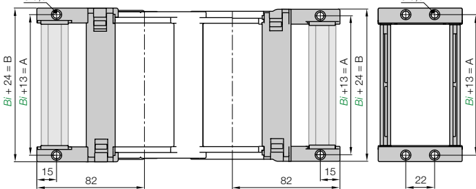
Variante KMA, pendelnd für E-Ketten® auf Anfrage
