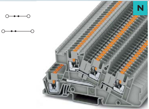
4 (4) mm², 30 A, Dreistockklemme, 2 x Außenleiter L
