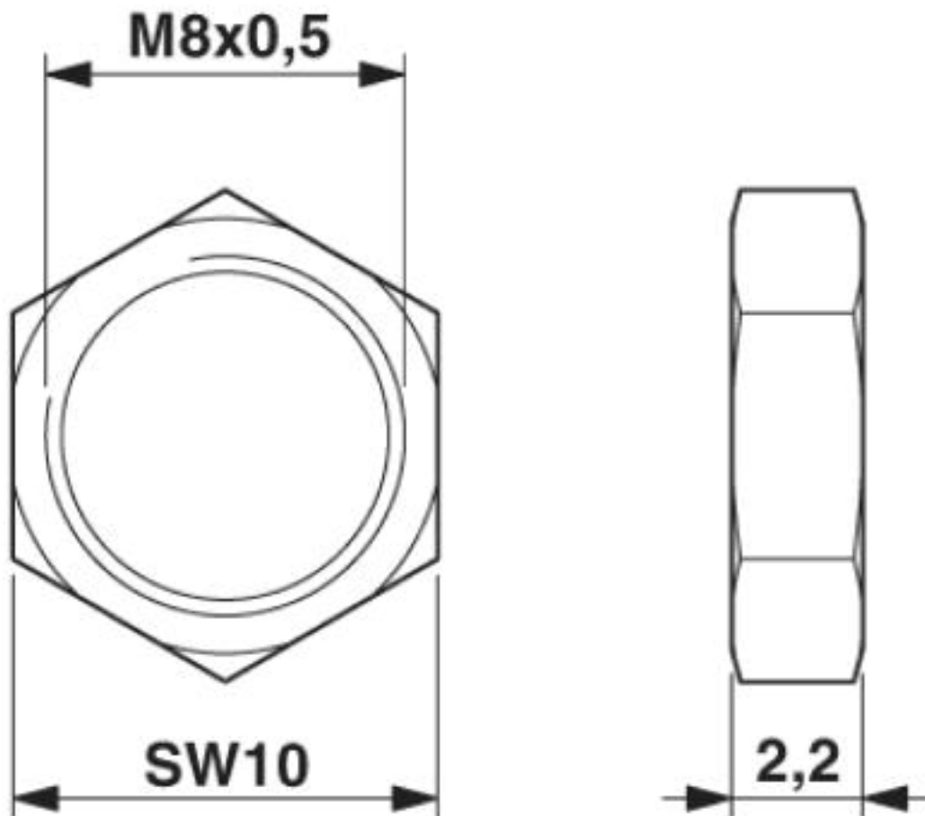
Flachmutter M8
