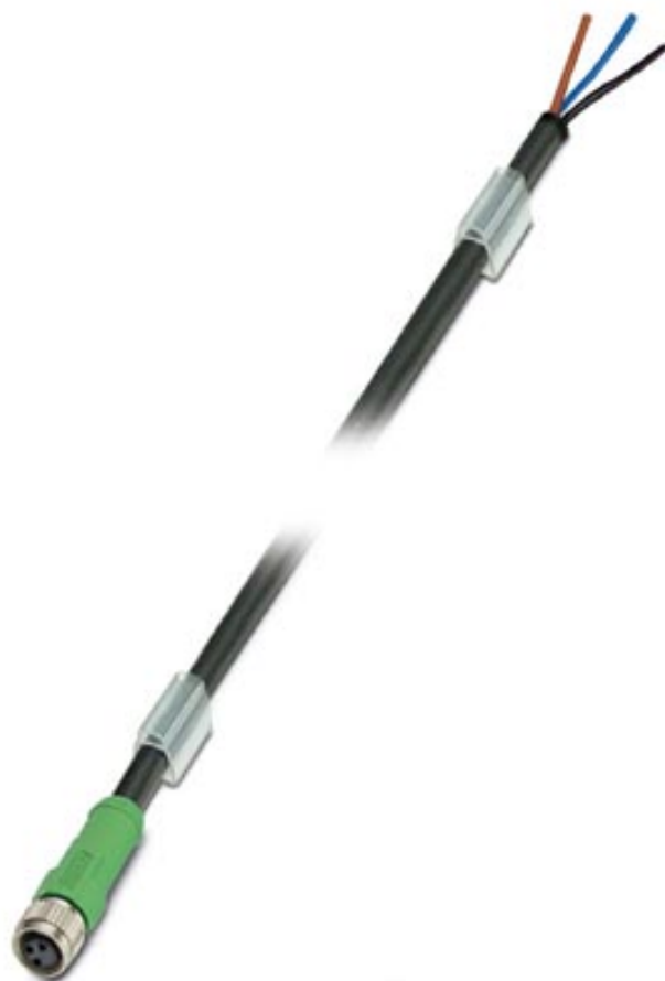
Sensor-Kabel, gerade Buchse M8, 4-polig, Kabellänge: 3 m
