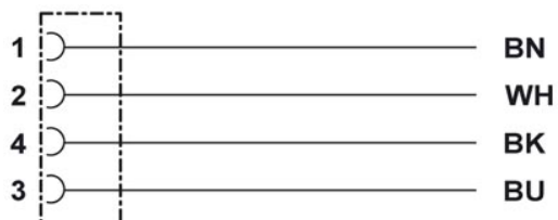
Kontaktbelegung der M8-Stecker/Buchsen
