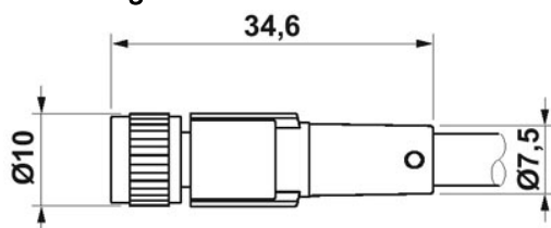
Buchse M8 x 1, gerade
