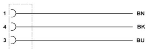
Kontaktbelegung der M12-Buchsen
