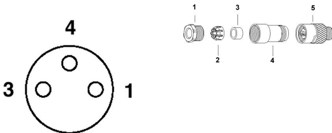
Schemazeichnung
