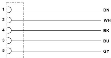
Kontaktbelegung der M12-Buchsen
