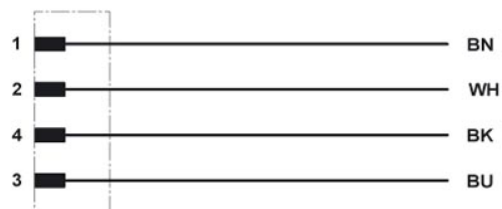
Kontaktbelegung der M12-Stecker
