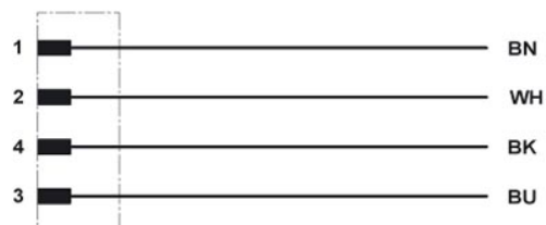
Kontaktbelegung der M12-Stecker / Buchsen
