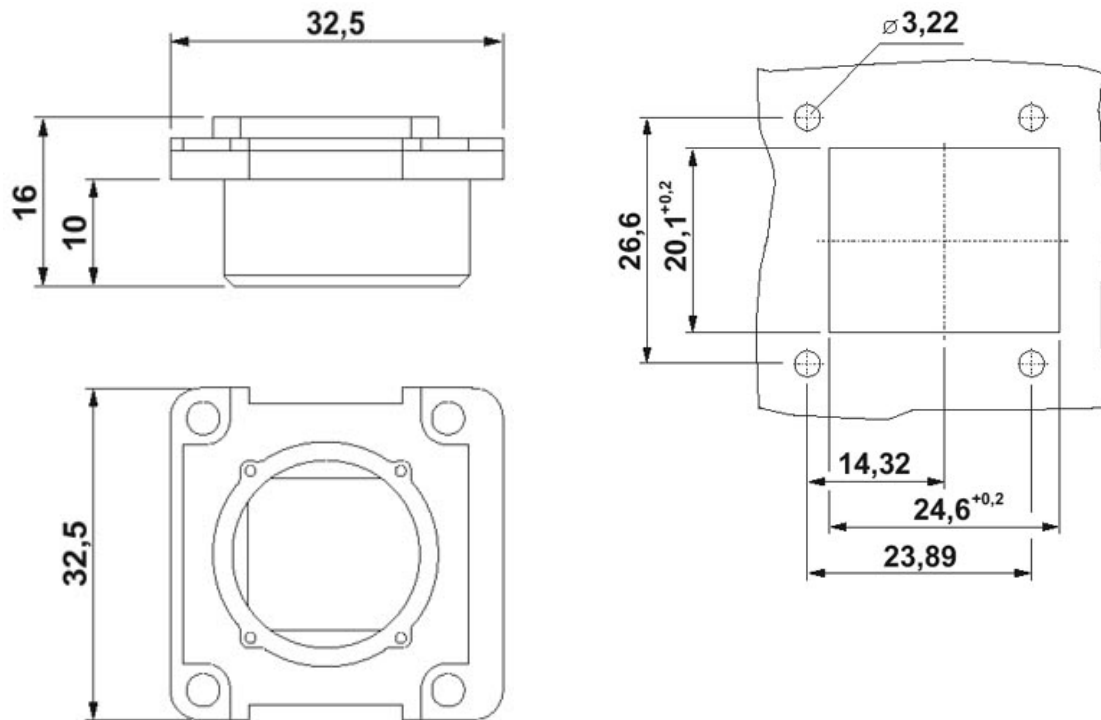
Montageausschnitt
