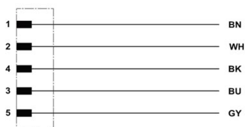
Kontaktbelegung der M12-Stecker
