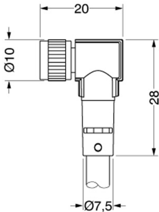
Maßzeichnung
