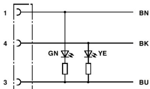
Schaltplan
