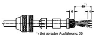
Absolieren, Schirm aufweiten und um den Schirmring legen, überstehendes Geflecht abschneiden.
