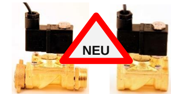
Magnetventile GMV 191-M-XX: Für ¾" Wasserhähne oder Rohrmontage
