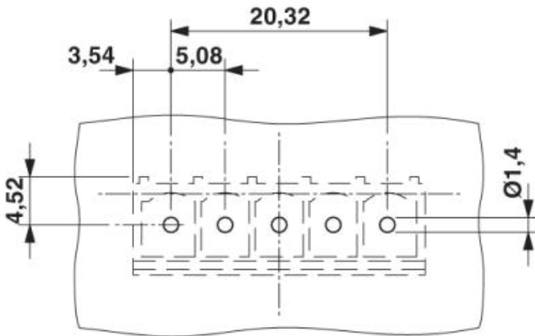
Bohrplan
