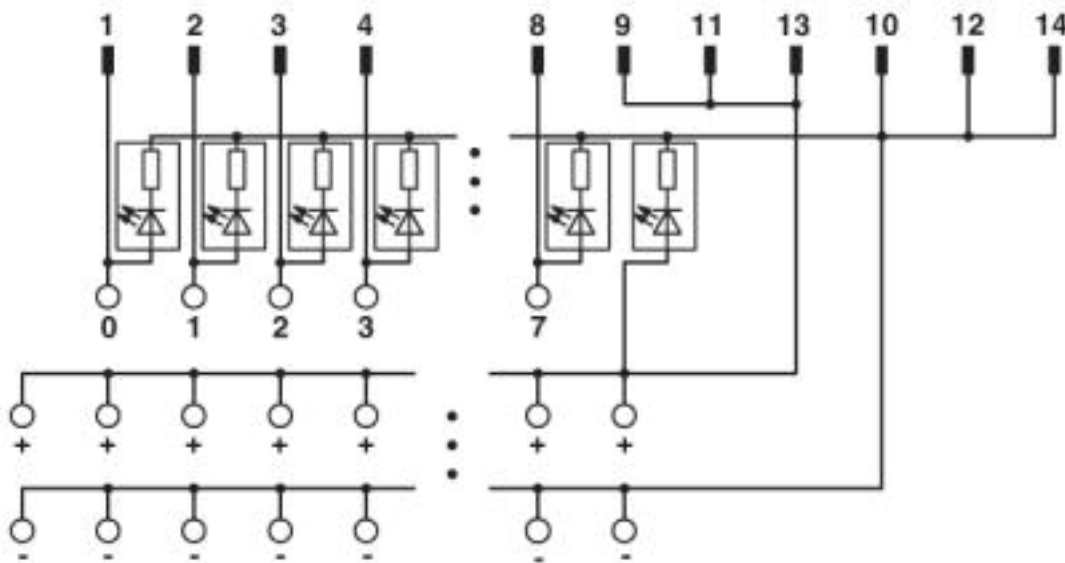
Anschlussbild FLKMS 14/8IM/LA/PLC
