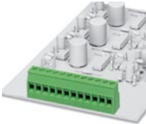
Leiterplattenklemme, Nennstrom: 24 A, Nennspannung: 400 V, Rastermaß: 5,08 mm, Polzahl: 2, Anschlussart: Schraubanschluss, Montage: Löten, Anschlussrichtung Leiter/Platine: 0 °, Farbe: grün
