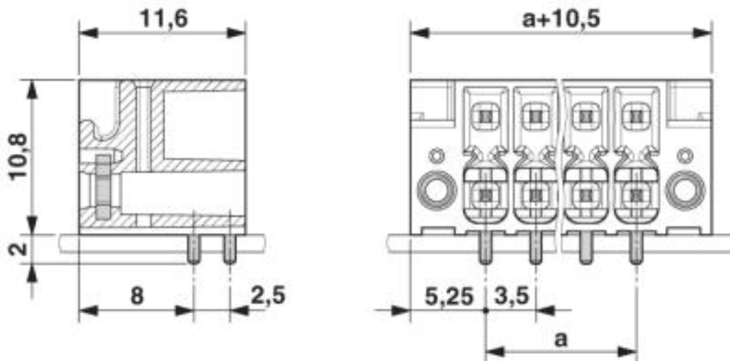
Maßzeichnung
