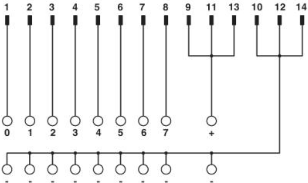
Anschlussbild VIP-2/.../FLK14/8M/PLC
