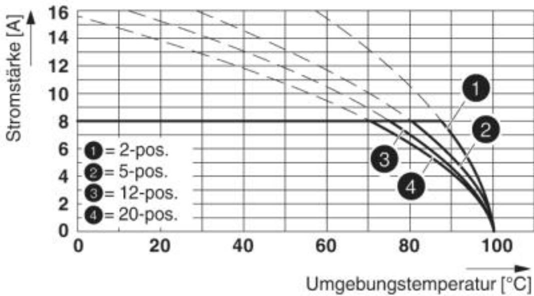
Typ: MC 1,5/...-STF-3,81 mit MC 1,5/...-GF-3,81
