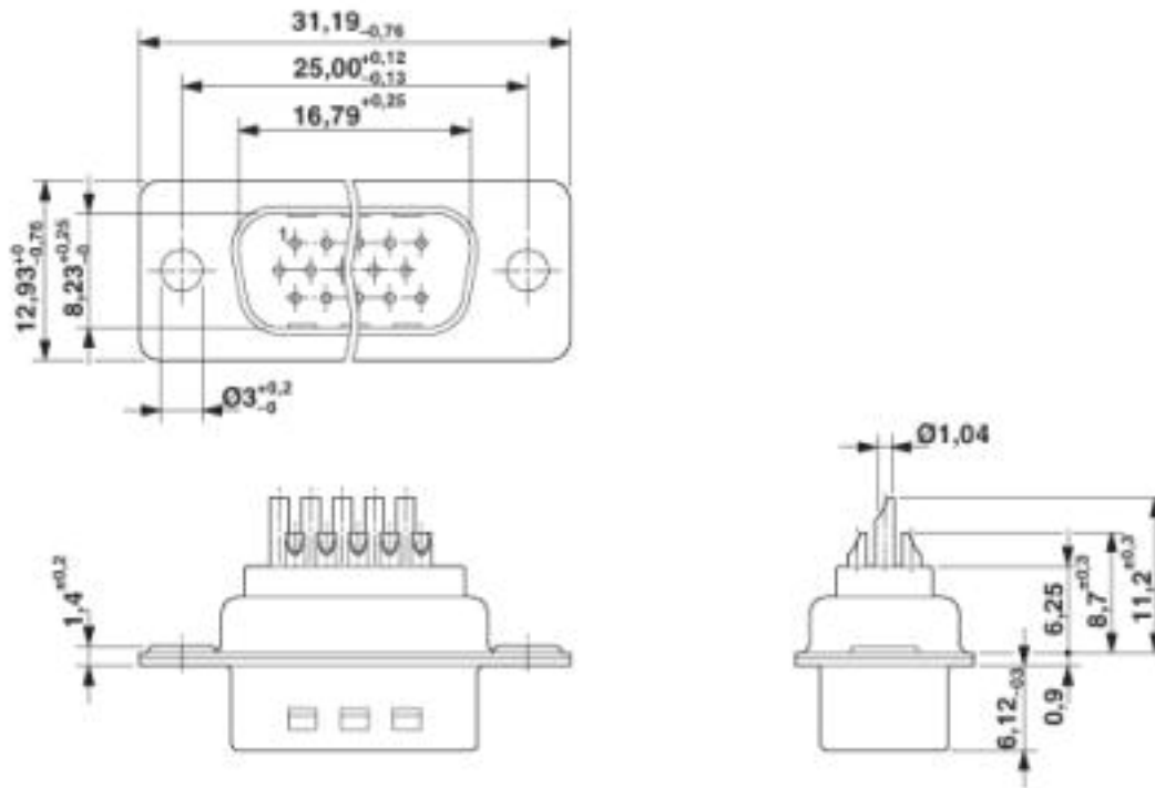
D-SUB Kontakteinsatz
