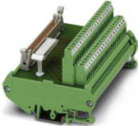
VARIOFACE-Übergabemodul, für MODICON® TSX Quantum, mit MODICON®-spezifischer Beschriftung, für Ein-/Ausgabe von 32 Kanälen
