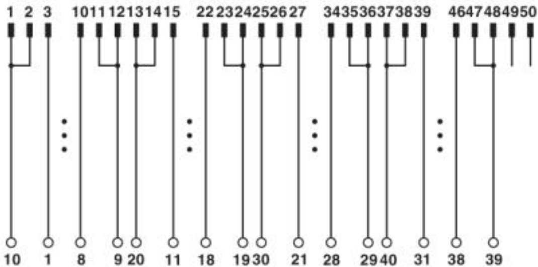
Anschlussbild FLKM 50/MODI-TSX/Q
