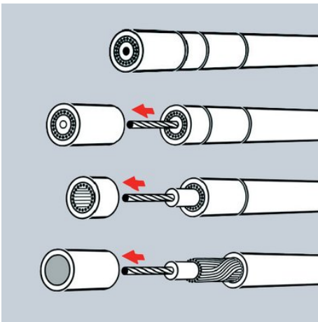
Dreistufige Abisolierung eines Koaxialkabels
