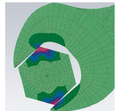
Herkömmlicher Schraubenschlüssel: Kantenpressung führt zu Beschädigung
