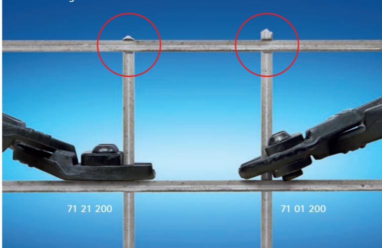
Schnitt mit Modell 71 21 200: fast bündiges Gitterende
