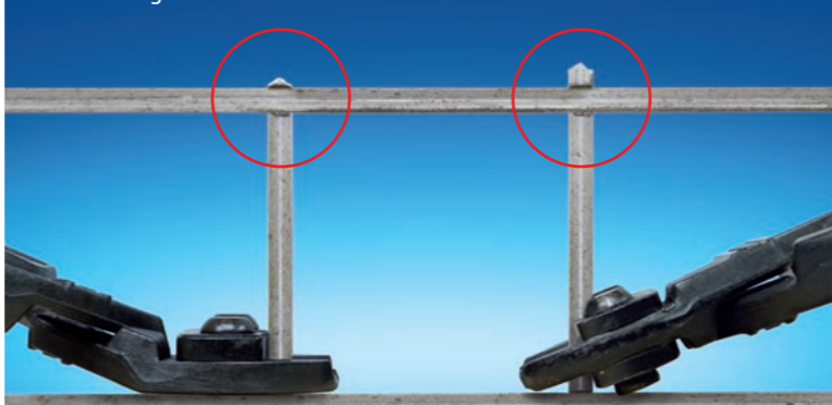
Schnitt mit Modell 71 21 200: fast bündiges Gitterende
