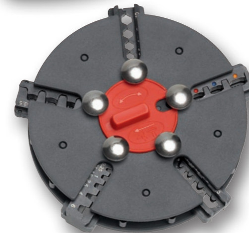
97 33 02 Crimpzange mit Rundmagazin und 5 Wechselseinsätzen für unisolierte, offene Steckverbinder; isolierte Kabelschuhe + Steckverbinder; Aderendhülsen; unisolierte Kabelschuhe + Steckverbinder; unisolierte Stoßverbinder
