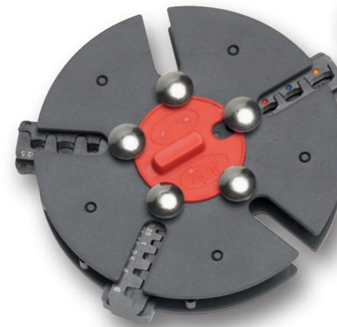
97 33 01 Crimpzange mit Rundmagazin und 3 Wechselseinsätzen für unisolierte, offene Steckverbinder; isolierte Kabelschuhe + Steckverbinder; Aderendhülsen
