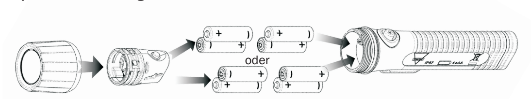
Bild 4: Explosionszeichnung PetaLux Typ 4910... mit Batterien
