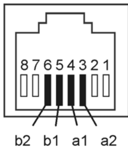
RJ-45-Buchse
