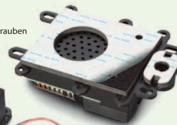
Mikrofongehäuse kann abgetrennt und separat angeschraubt/angeklebt werden
