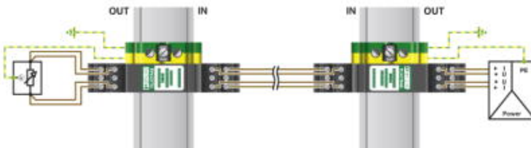
Applikationszeichnung
