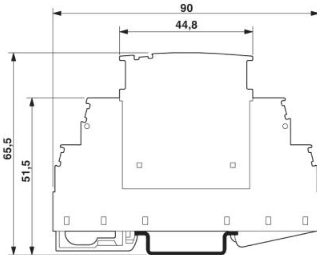
Maßzeichnung
