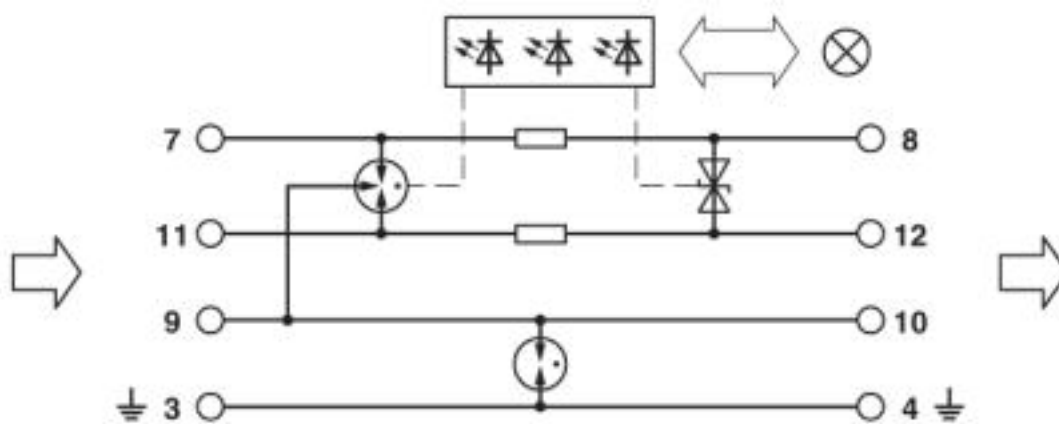
Schaltplan
