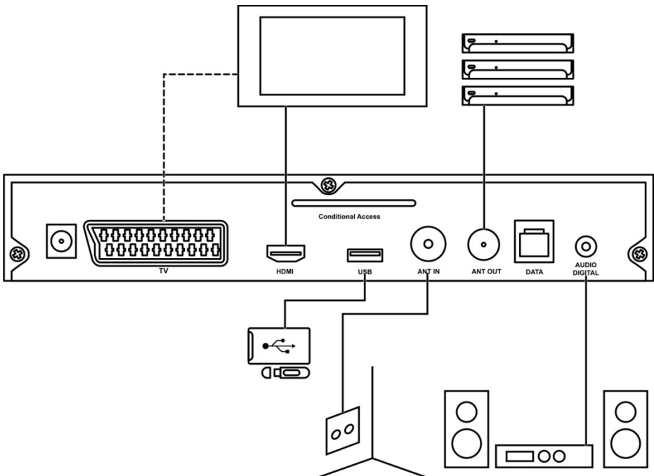
Abbildung 3: Anschluss-Schema
