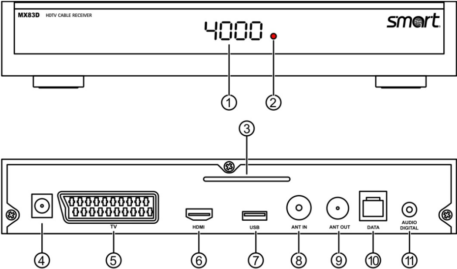
Abbildung 1: Bedienelemente und Anschlüsse
