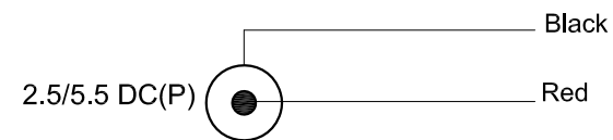
Wiring
