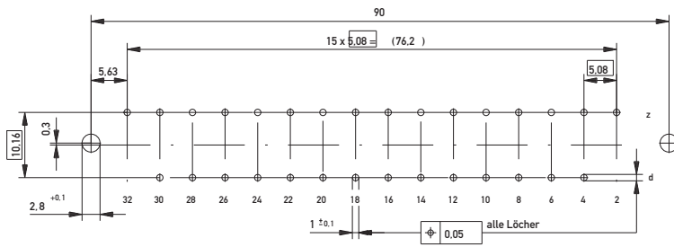
Leiterplatten-Lochbild
