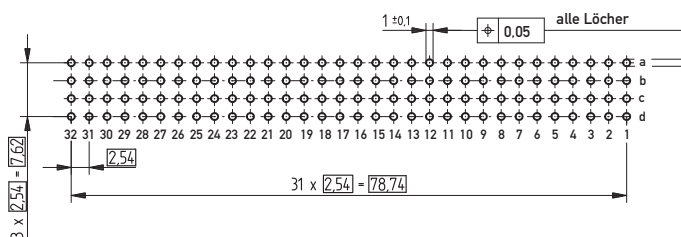
Leiterplatten-Lochbild
