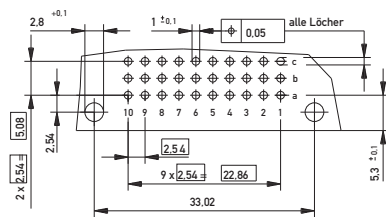
Leiterplatten-Lochbild
