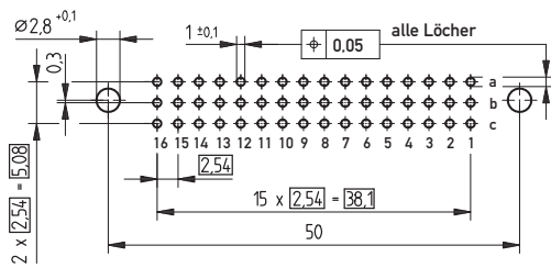
Leiterplatten-Lochbild
