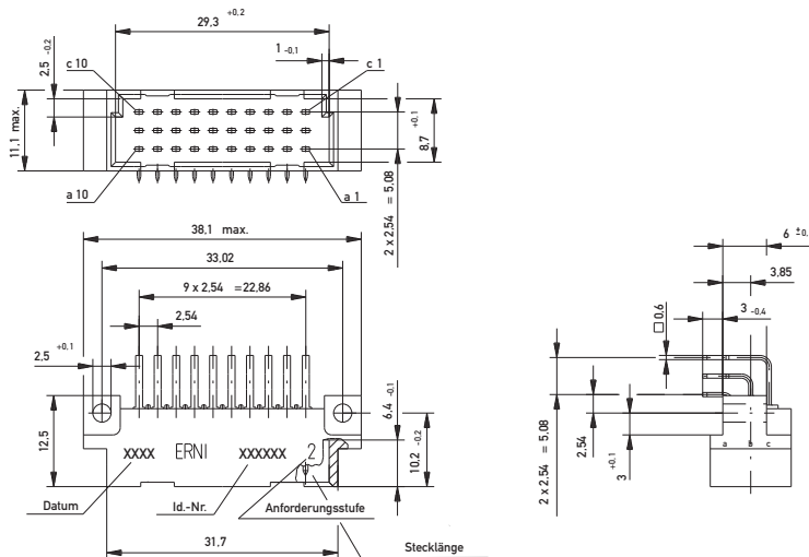
Leiterplatten-Lochbild
