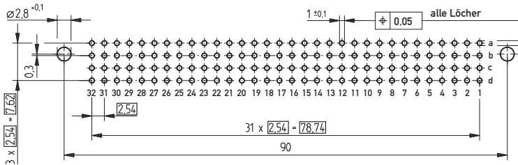
Leiterplatten-Lochbild
