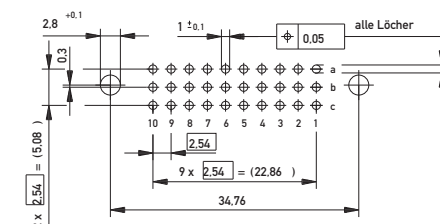
Leiterplatten-Lochbild
