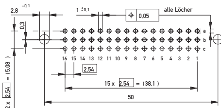
Leiterplatten-Lochbild
