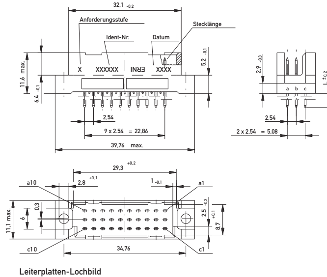
Leiterplatten-Lochbild
