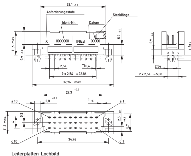
Leiterplatten-Lochbild
