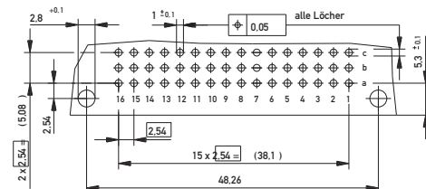
Leiterplatten-Lochbild
