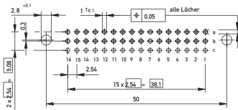
Leiterplatten-Lochbild
