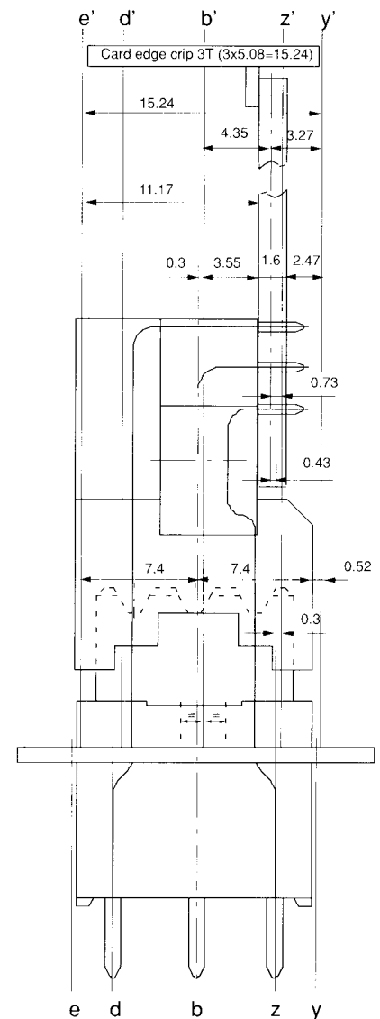
Exakte Position der Steckverbinder Bauform F
