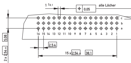
Leiterplatten-Lochbild
