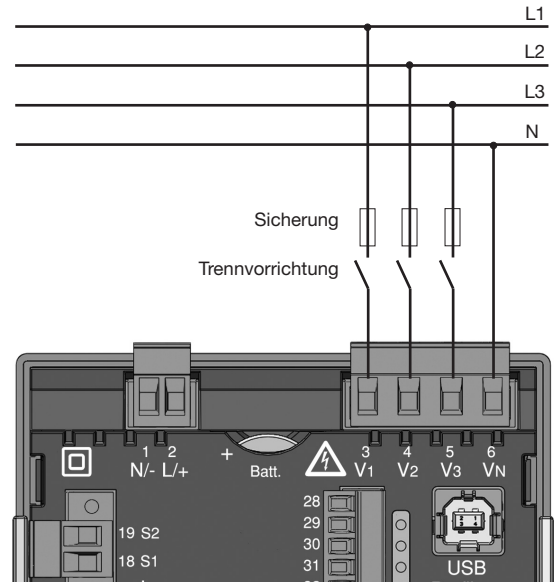
Abb. Anschlussbeispiel für die Spannungsmessung
