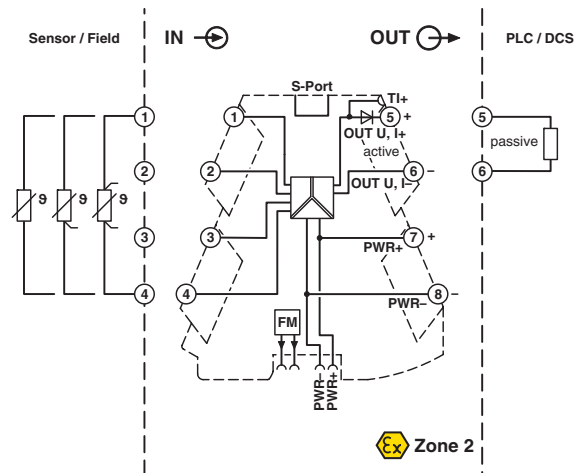
Bild 2 Blockschaltbild
