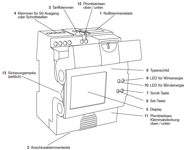
Funktionselemente
