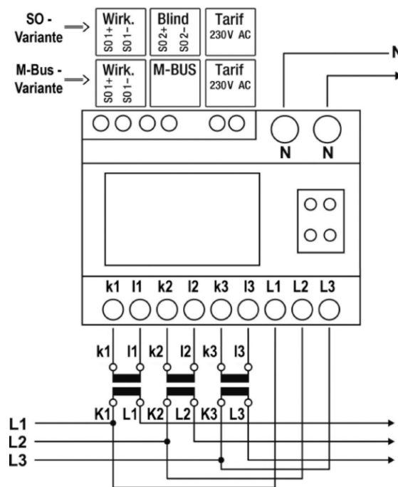
Anschlussschaltung
