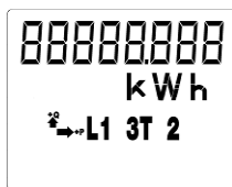
keine Spannung an L2
